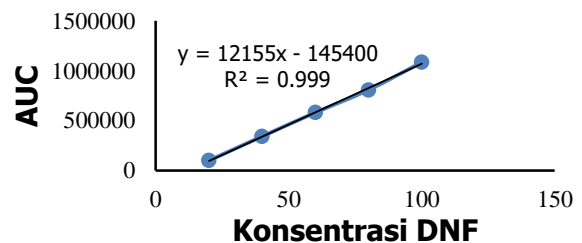
Gambar 2. Kurva hubungan antara konsentrasi deksametason natrium fosfat dan AUC
