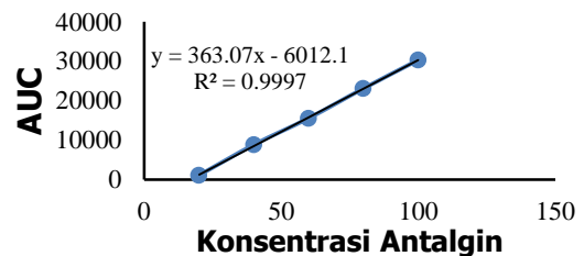
Gambar 1. Kurva hubungan antara konsentrasi antalgin dan AUC
