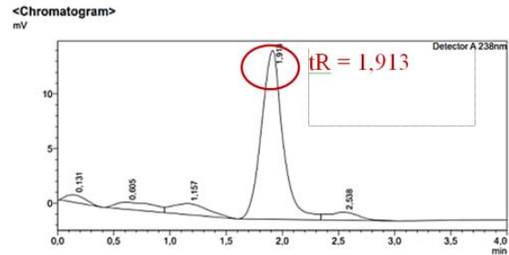
Gambar 4. Kromatografi sampel mengandung deksametason natrium fosfat
