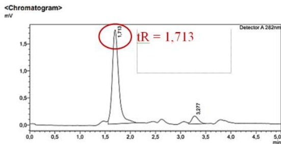
Gambar 3. Kromatografi sampel mengandung antalgin
