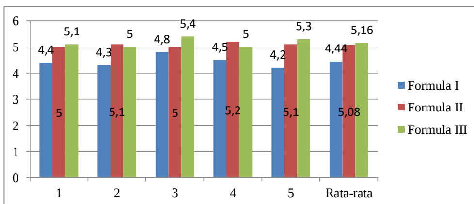
Gambar 4 Grafik Evaluasi Uji Kekerasan (Data diolah, 2021)
