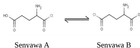
Gambar 4.7 Struktur Kimia Hasil Sintesis
