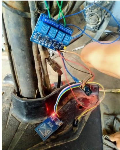
Gambar 5. Pengaplikasian Modul Ke Sepeda Motor Matic
