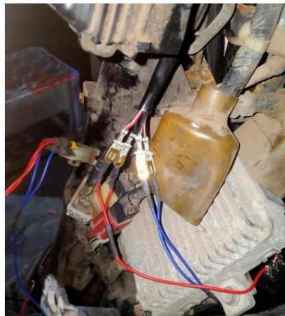
Gambar 4. Pengaplikasian Modul Ke Sepeda Motor Matic
